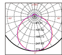
NPXLED1008 24W 120°
